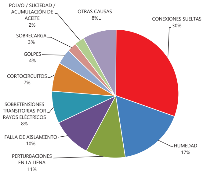
Principales causantes de falla en sistemas de Distribución Eléctrica
